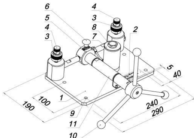
Рисунок 1- Пресс ПГ 700/1000/
